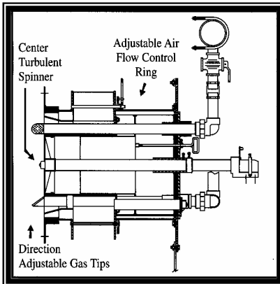
KE Low NOx Burner
